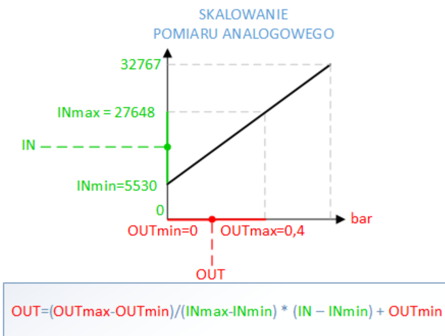
Rys. 3.6 Charakterystyka przetwornika laboratoryjnego ciśnienia
