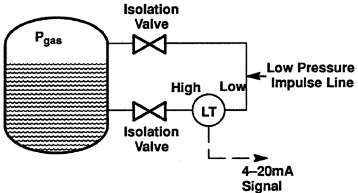
Rys. 5 Zdalny pomiar poziomu cieczy zbiornika zamkniętego za pomocą przetwornika różnicy ciśnień.
