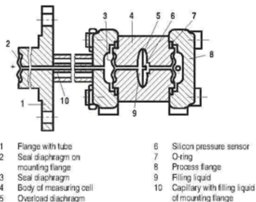
Rys. 7 Schemat elektronicznego przetwornika różnicy ciśnień z rysunku 6.
