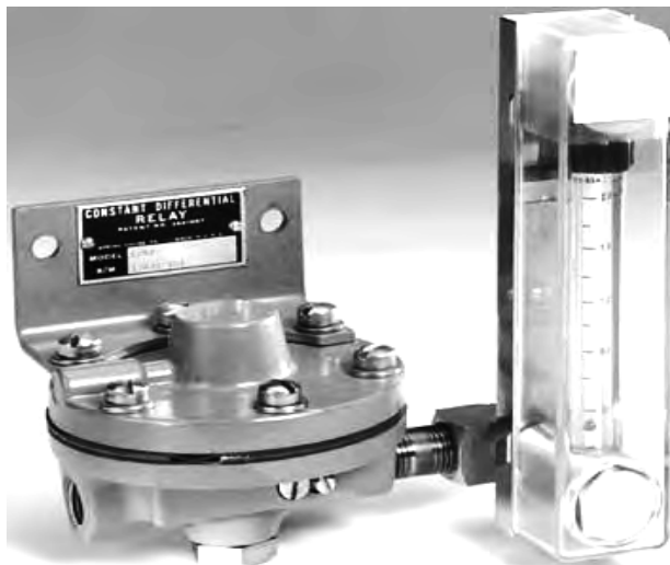
Rys. 11 Regulator małych przepływów, a-widok zewnętrzny regulatora z widocznym zaworem iglicowym, b-zespół regulatora z rotametrem.
