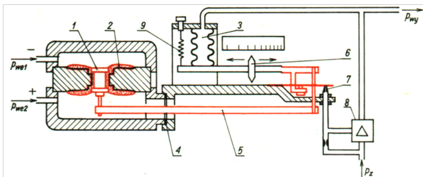
Rys. 8 Mechaniczno-pneumatyczny przetwornik różnicy ciśnień.
