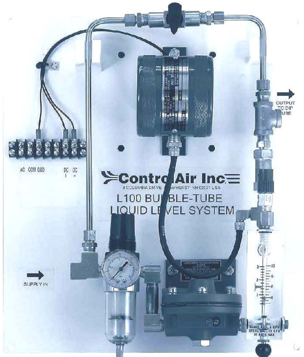
Rys. 12 Pełny zestaw pomiarowy sondy bąbelkującej do pojedynczego zbiornika firmy ControlAir.
