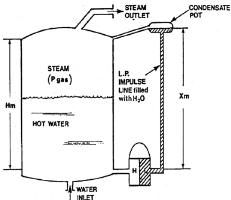
Rys. 6 Pomiar poziomu wody w kotle oraz wskaźnik poziomu wody oparty o przetwornik różnicy ciśnień.
