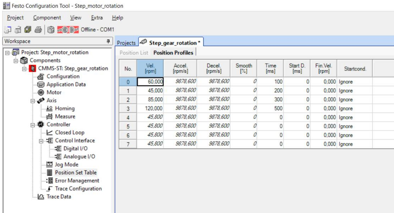
Rys. 4.17 Tablica rekordów z określeniem parametrów ruchu w programie FCT
