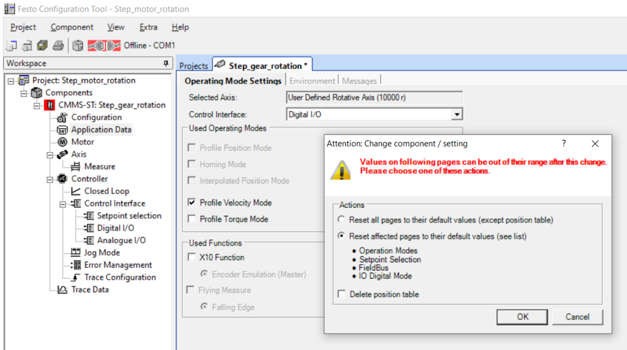
Rys. 4.12 Włączenie pozycjonowania, sygnał analogowy
