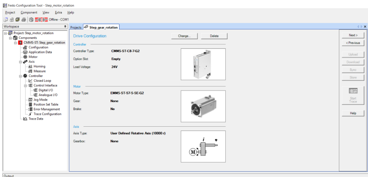
Rys. 3.10 Wprowadzone parametry konfiguracyjne układu napędowego
