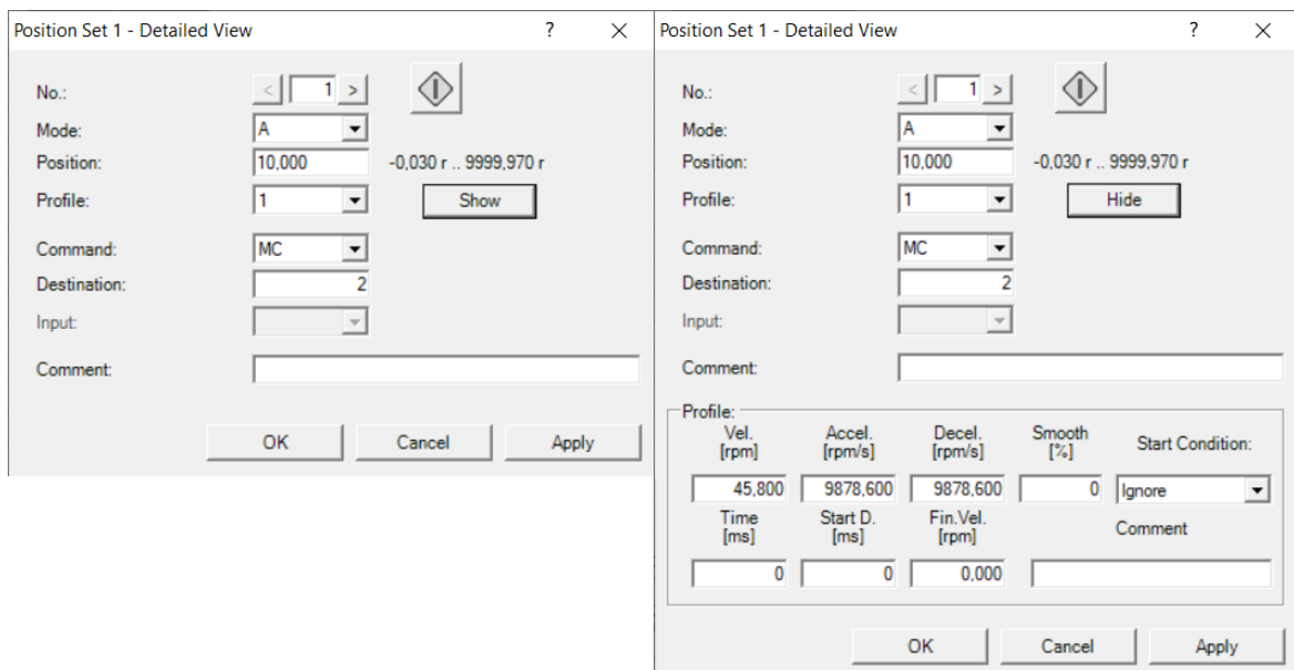
Rys. 4.18 Okno dialogowe z parametrami pozycji i ruchu w programie FCT
