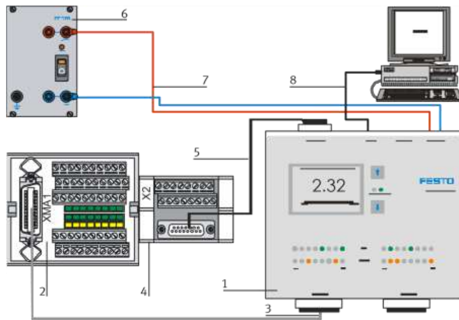
Rys. 2.4 Zasilanie układu
