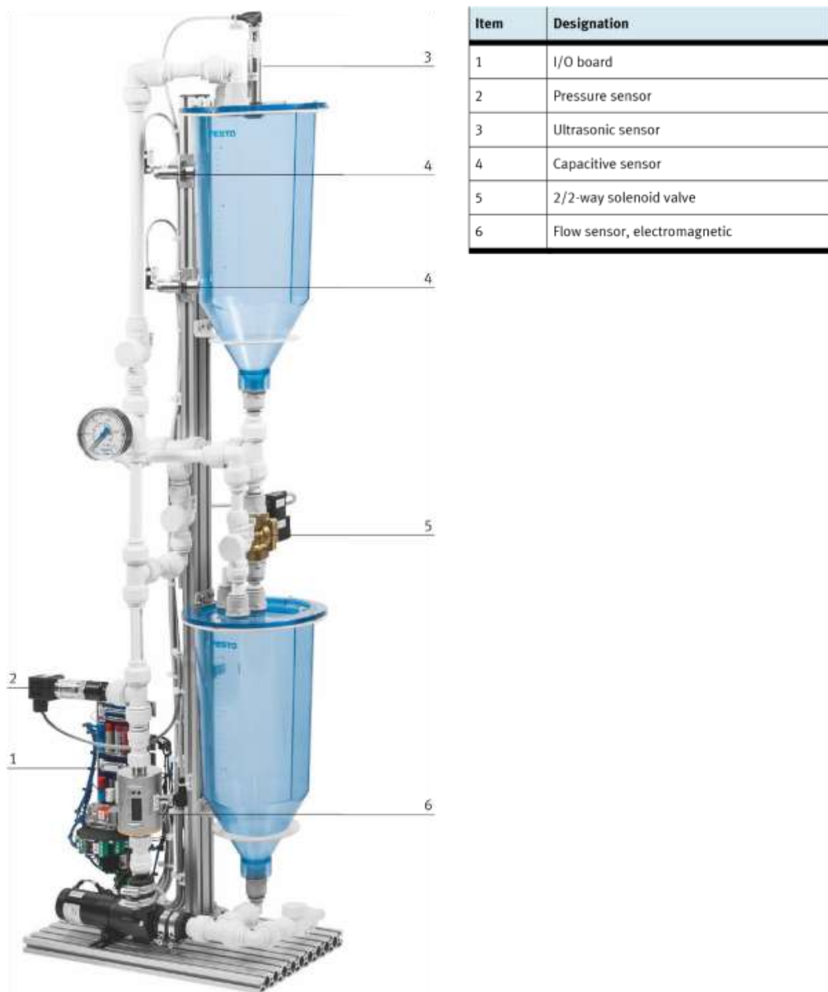
Rys. 2.2 Stanowisko z układem pompowym do badania charakterystyk członu całkującego
