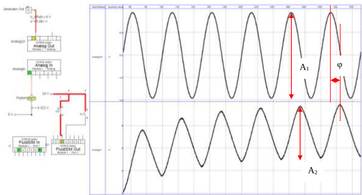
Rys. 4.9 Odczyt parametrów dla f = 0.02\text{Hz} ; A_1 = 2\text{V} , A_2 = 2.1\text{V} , \varphi = 12.5\text{s} to jest 90^\circ
