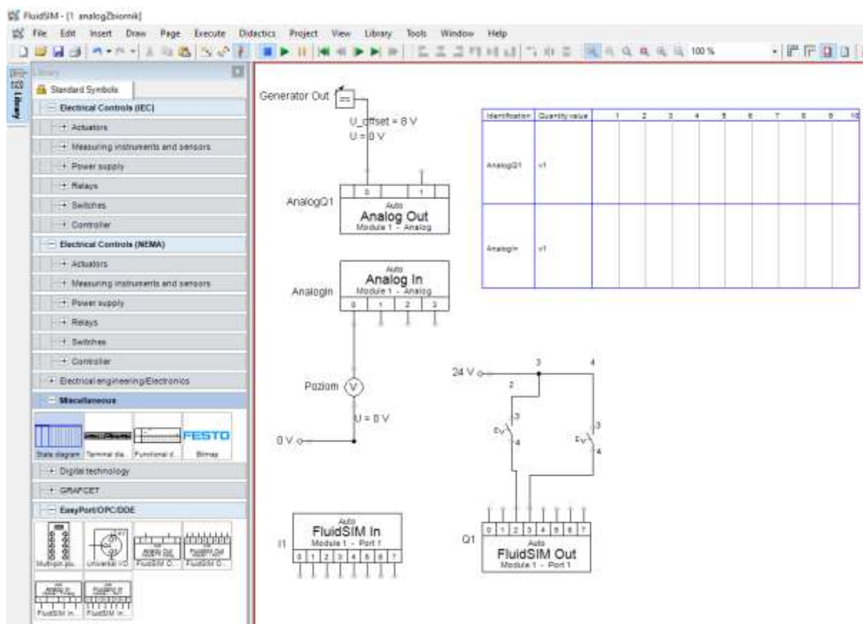
Rys. 3.9 Program we FluidSIM do rejestracji charakterystyk dynamicznych układu pompowego
