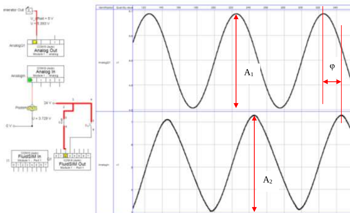
Rys. 4.8 Odczyt parametrów dla f = 0.01\text{Hz} ; A_1 = 2\text{V} , A_2 = 4.2\text{V} , \varphi = 25\text{s} to jest 90^\circ
