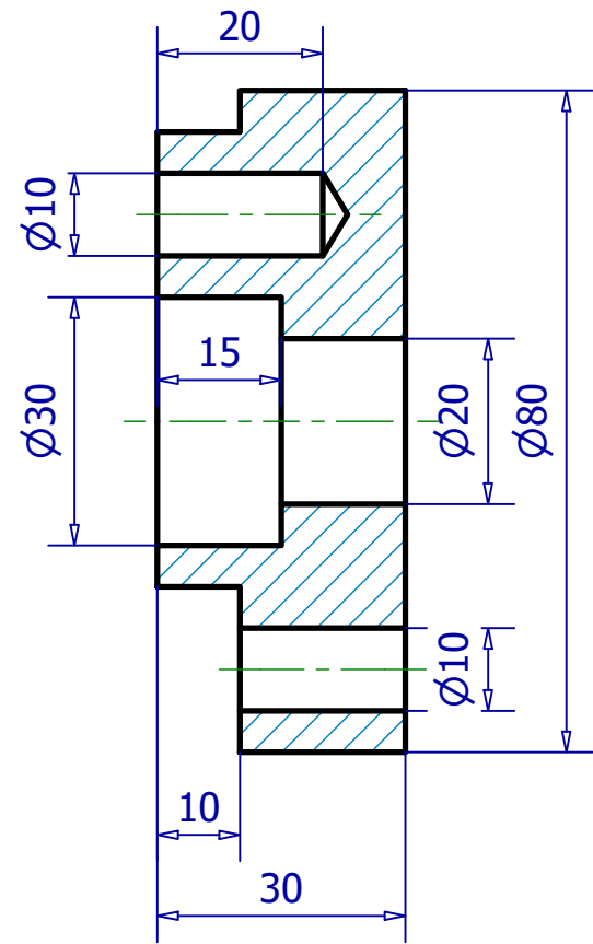
A-A ( 1 : 1 )
